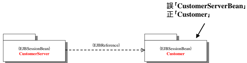
図2.8 UML Profile for EJBを用いて記述した例3 (内部ビュー)
