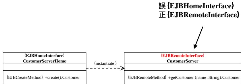
図2.6 UML Profile for EJB を用いて記述した例1 (外部ビュー)
